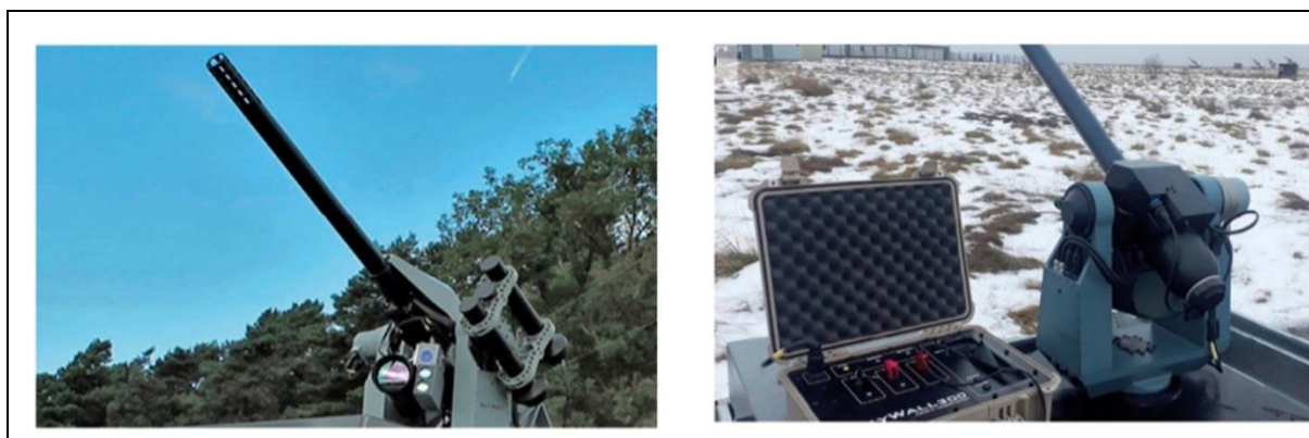
Рис. 3 - Пневматическая турель для запуска снаряда с противодронной сетью-ловушкой
